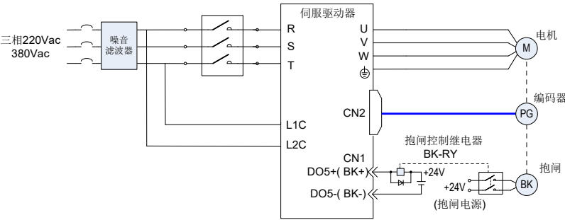
图 3-15 抱闸配线图
