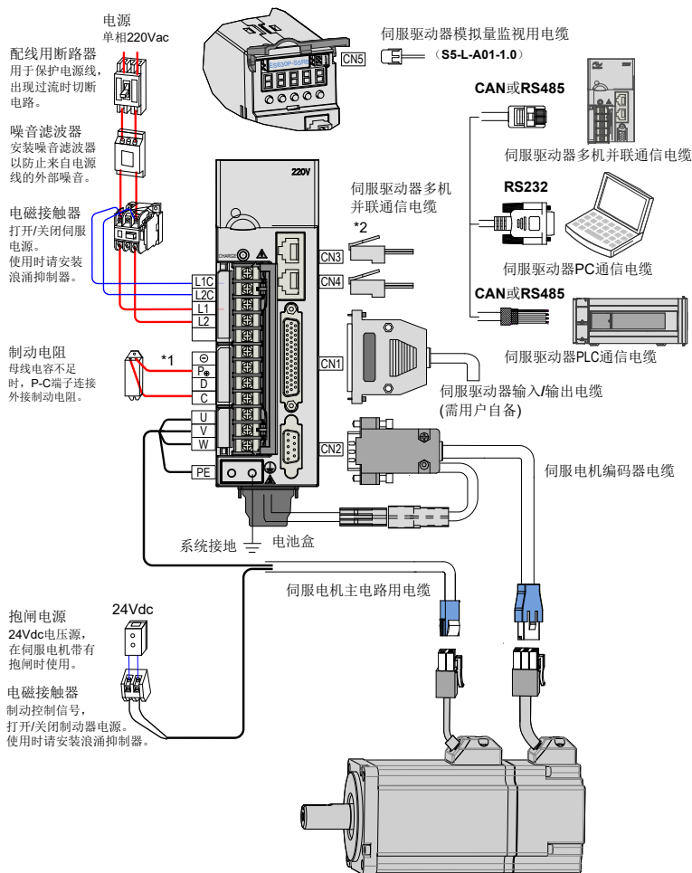
图 1-2 单相 220V 系统配线图举例
