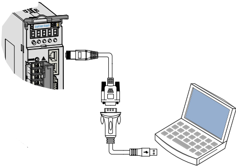
图 3-28 通信串口转 USB 示意图
