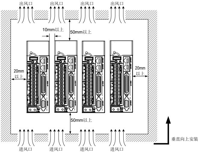
图 2-1 伺服驱动器安装示意图
