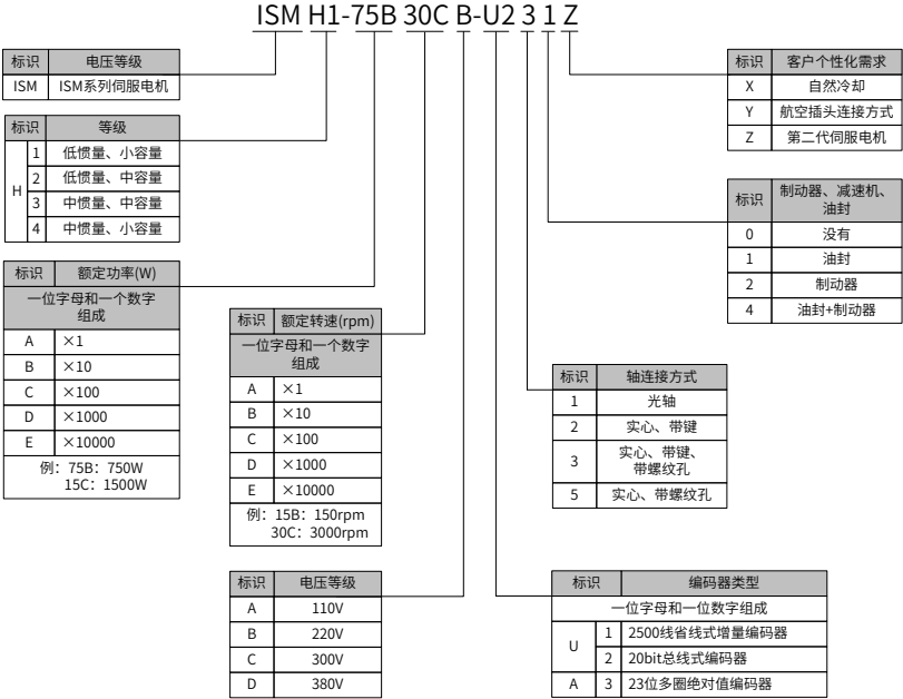
图 1-3 伺服电机型号说明
