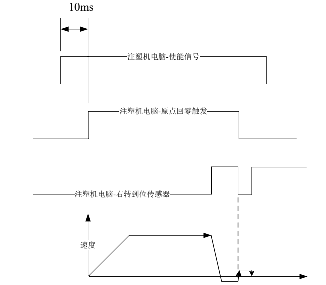
图 5-4 回零时序图
