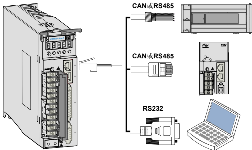
图 3-18 通信配线示意图
