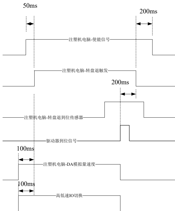
电脑端子时序图
