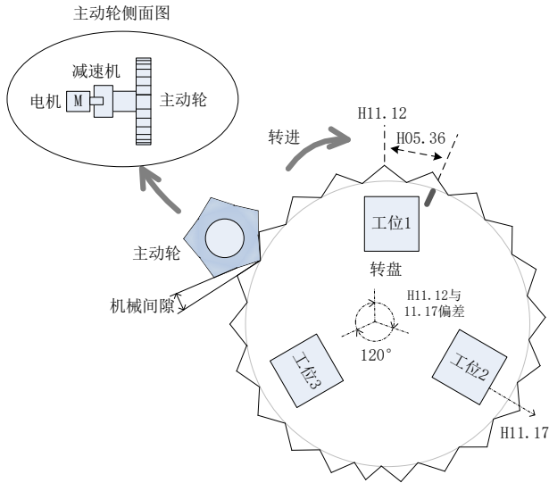
图 5-2 三工位机器工作示意图
