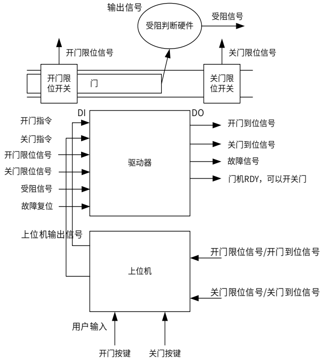
图 B-1 门机方案
