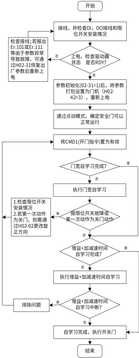
图 B-2 门机调试流程图
