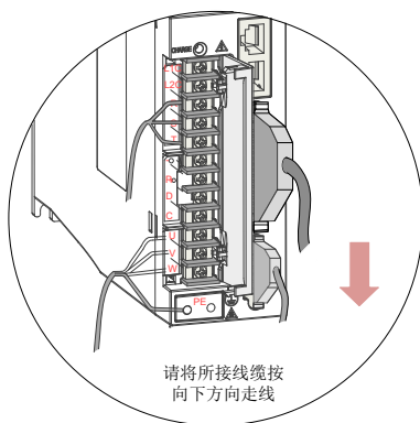
图 2-2 伺服驱动器线缆走线要求示意图
