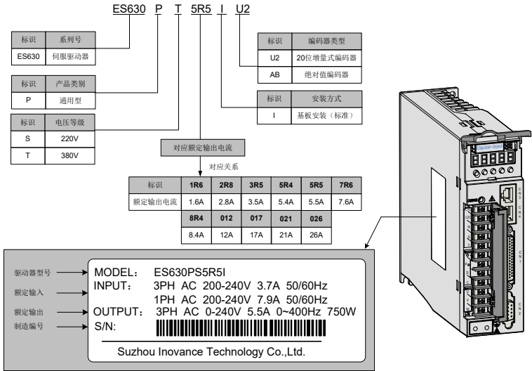
图 1-4 伺服驱动器型号说明
