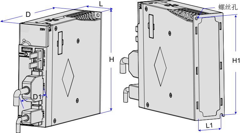
图 2-3 驱动器尺寸图
