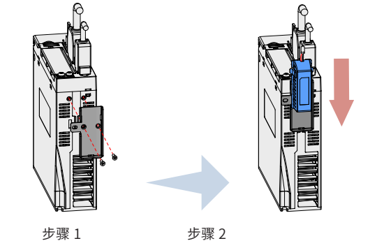
图 3-9 绝对值编码器电池盒安装示例图（sizeA 机型，仰视图）
