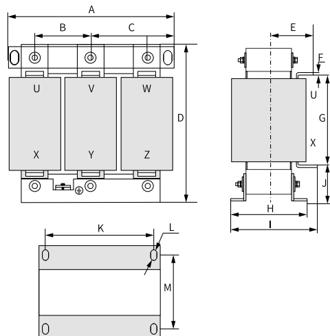
图6-14 150A~250A交流输出电抗器尺寸图
