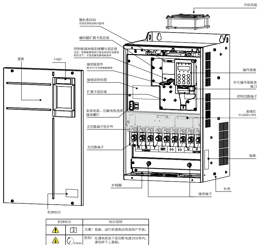
图1-4 产品部件示意图 (T7~T9)
