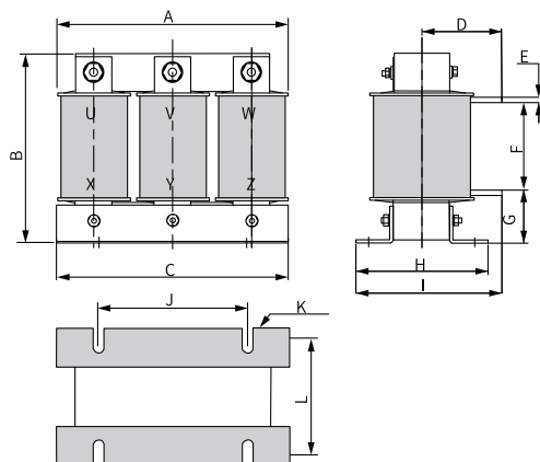
图6-13 80A~120A交流输出电抗器尺寸图
