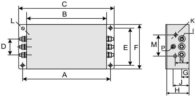
图6-9 强力滤波器（50A~200A）尺寸图
