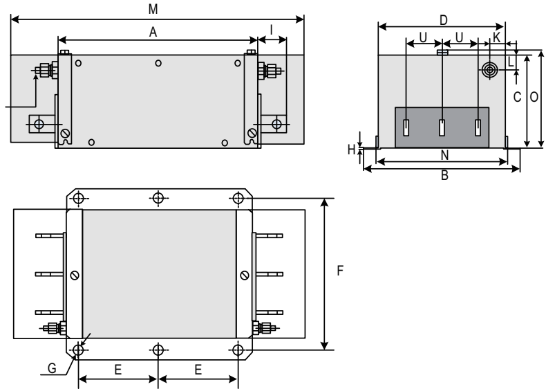
图6-7 FN 3359系列滤波器（320A~2500A）尺寸图
