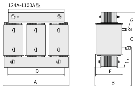
图6-18 输出电抗器尺寸图（124A~330A）
