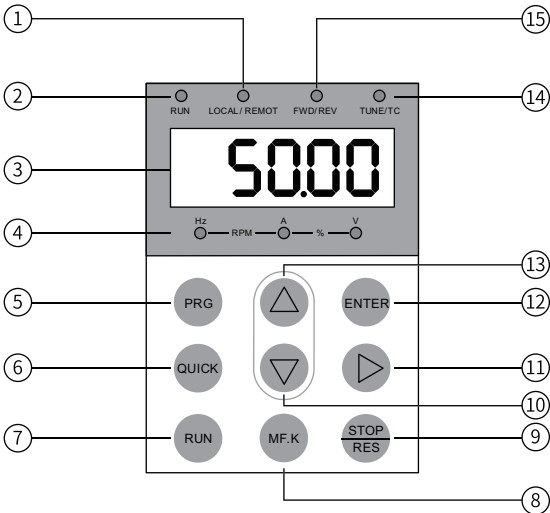
图3-1 部件示意图
