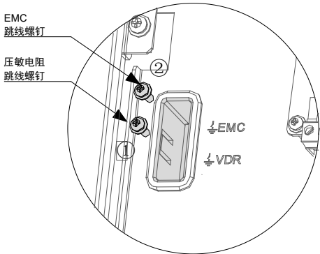
图 2-19 压敏电阻（VDR）、安规电容（EMC）对地跳线位置示意图
