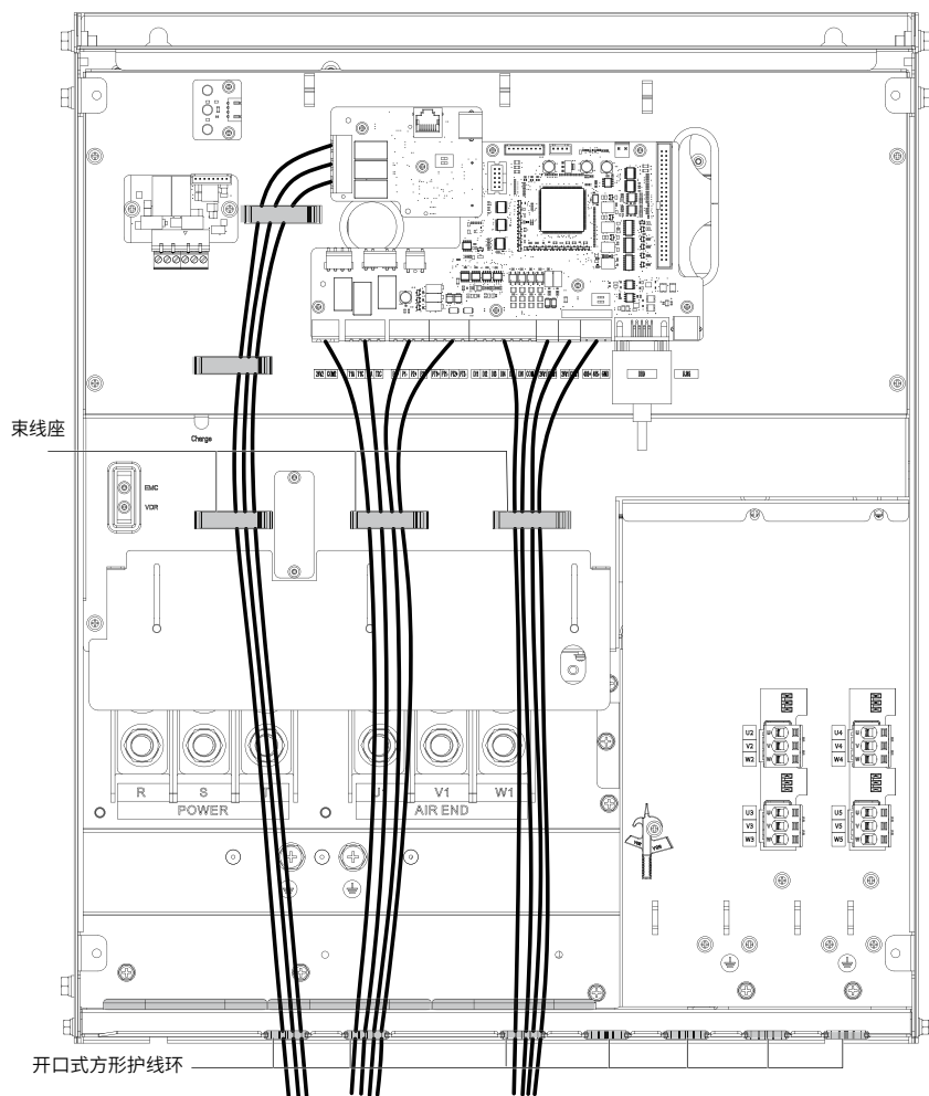
图 2-24 控制线线缆走线示意图 (CP700-4T110-H~CP700-4T200-H、CP700-4T110-H.7.5~CP700-4T200-H.7.5 机型)
