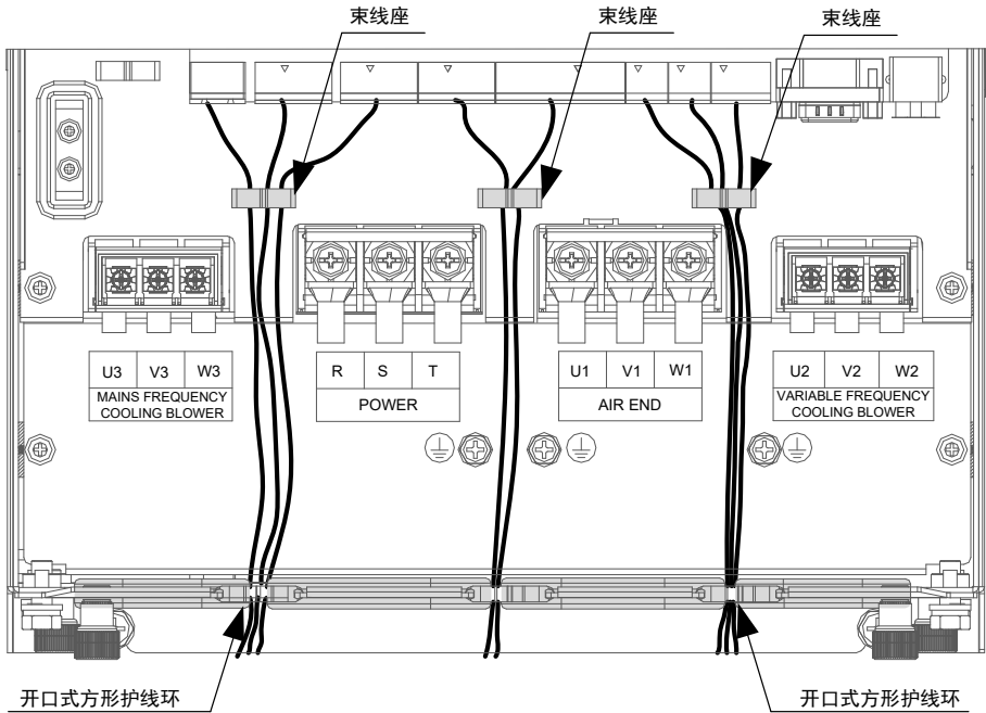
图 2-23 控制线线缆走线示意图 (CP700-2T7.5-H~CP700-2T45-H 以及 CP700-4T5.5-H~CP700-4T90-H 机型)
