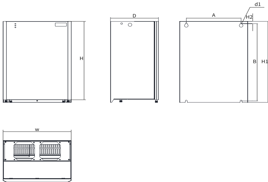
图 1-6 壁挂式安装尺寸图 (CP700-4T45-H~CP700-4T90-H)
