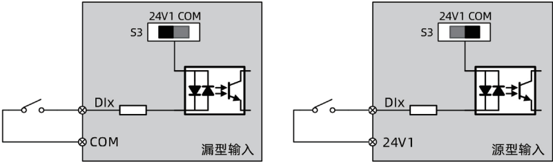
图 2-18 数字输入端子源型漏型接线示意图
