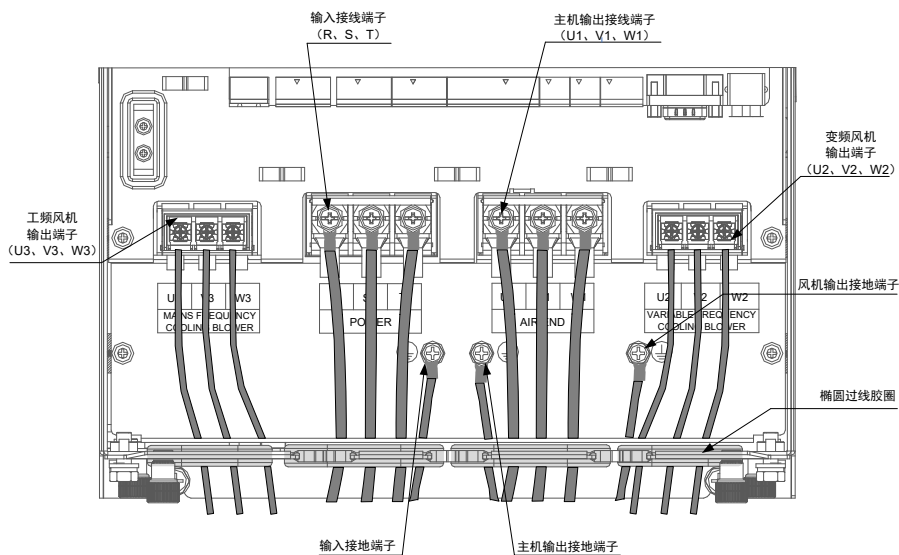
图 2-20 主功率线接线示意图 (CP700-2T7.5-H~CP700-4T90-H 机型)
