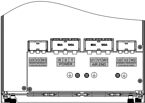
图 2-6 CP700-2T18.5-H~CP700-2T22-H、CP700-4T30-H~CP700-4T37-H 主回路端子分布示意图
