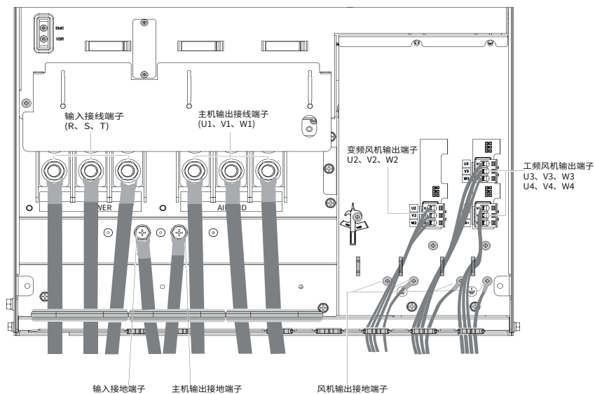
图 2-22 主功率线接线示意图 (CP700-4T110-H-7.5~CP700-4T200-H-7.5 机型)
