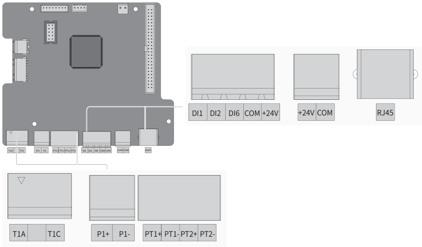
图 2-11 CP700-2T7.5-H 及 CP700-4T5.5-H~CP700-4T15-H 机型控制端子示意图
