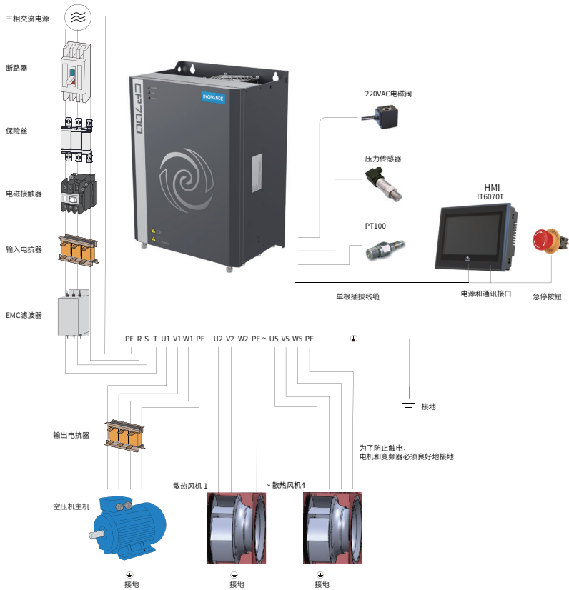
图 1-9 CP700 系统构成说明
