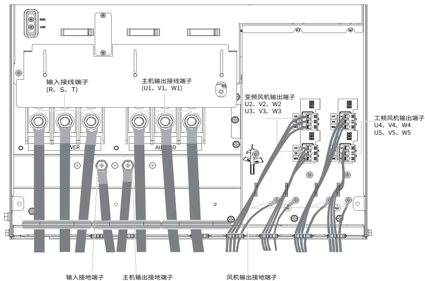
图 2-21 主功率线接线示意图 (CP700-4T110-H~CP700-4T200-H 机型)
